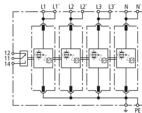
Prinzipialschaltbild DV M TNS 255 FM
