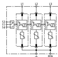
Prinzipialschaltbild DG M TNC 275 FM
