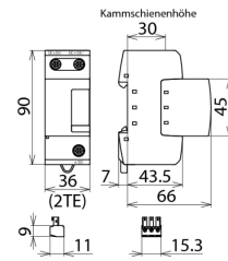
Maßbild DSE M 1 242 FM
