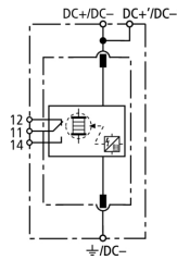
Prinzipialschaltbild DSE M 1 242 FM
