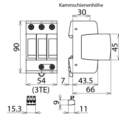
Maßbild DG M TNC 150 FM
