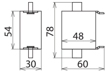
Maßbild DBM NH00 255
