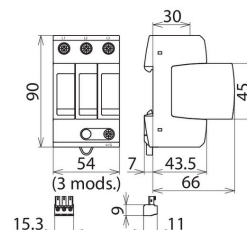
Maßbild DG MU 3PY 480 3W+G R
