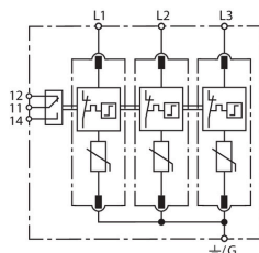
Prinzipialschaltbild DG MU 3PY 480 3W+G R
