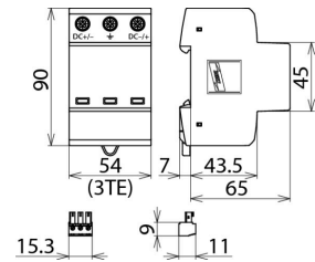
Maßbild DG YPV SCI 600 FM
