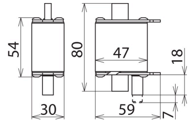
Maßbild VA NH00 280 FM
