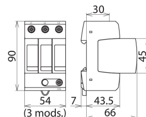
Maßbild DG MU 3PY 208 3W+G
