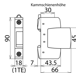
Maßbild DK 25
