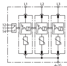
Prinzipialschaltbild DG MU 3PD 480 3W+G R
