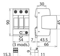
Maßbild DG MU 3PD 480 3W+G R
