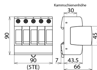
Maßbild DG M PV2 SCI 1000
