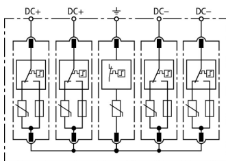
Prinzipialschaltbild DG M PV2 SCI 1000
