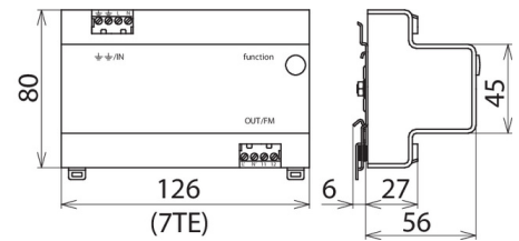
Maßbild SPS PRO
