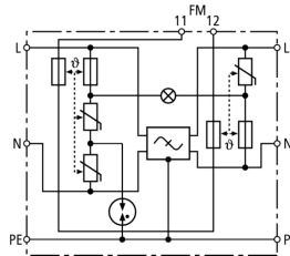
Prinzipschaltbild SPS PRO
