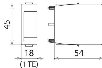
Maßbild DG MOD A NPE
