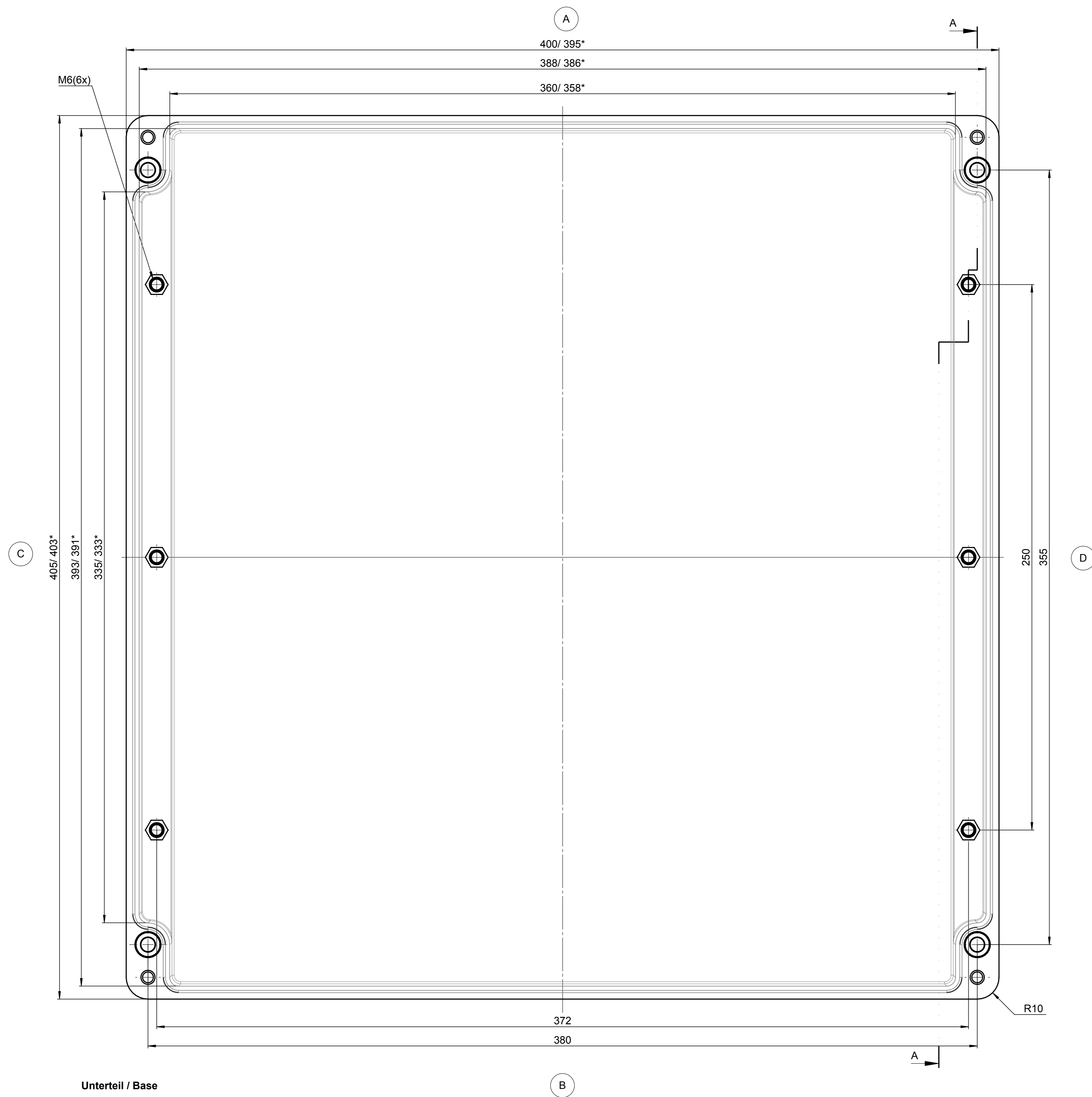
Unterteil / Base
