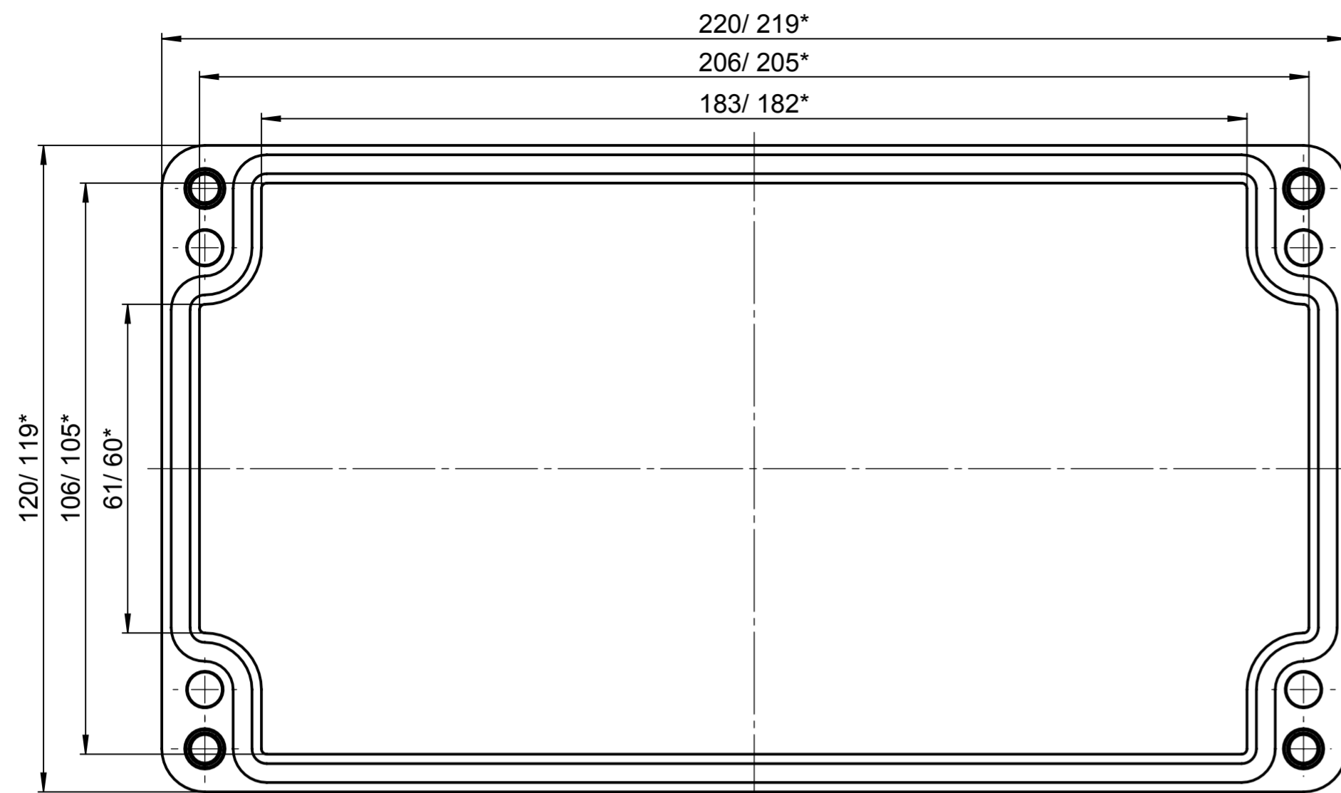
Deckel / Lid
