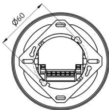
Bemaßung 92575
