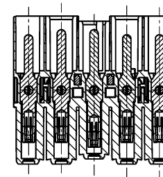
D-D
