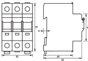
Maßzeichnung Gruppenansicht
