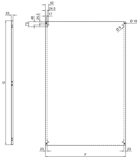
Montageplåt
