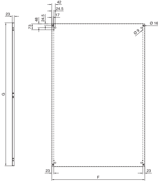
Montaj plakası
