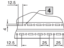
Delik şablonu
