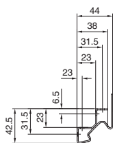
Przekrój profilu
