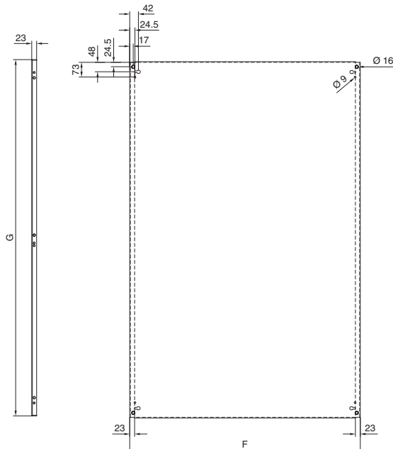
Płyta montażowa
