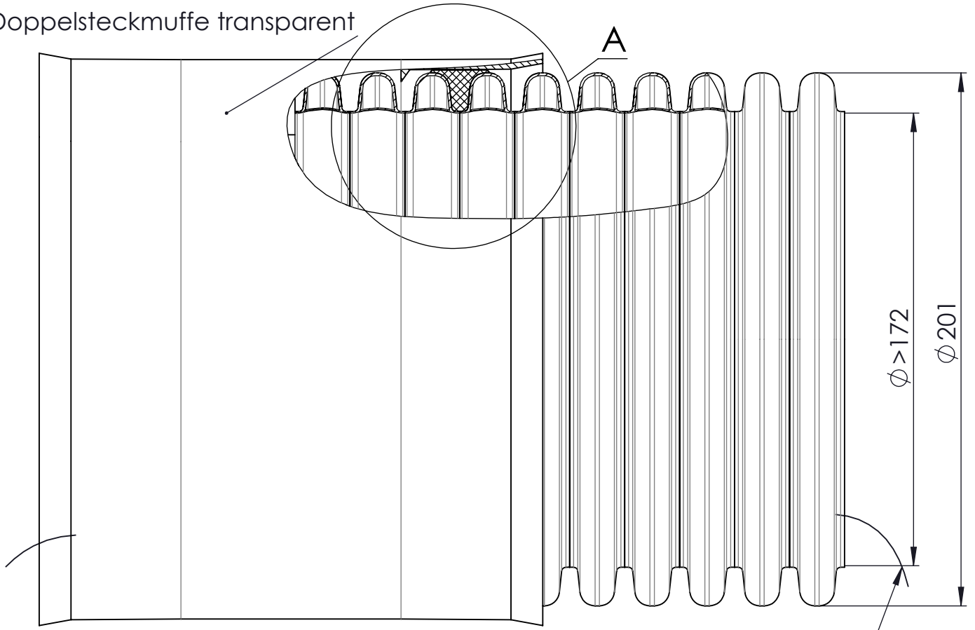
DETAIL A 1 : 1 optional mit Profildichtring montiert im 3. Wellental
