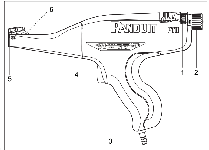
Pneumatisches Handwerkzeug PTH
