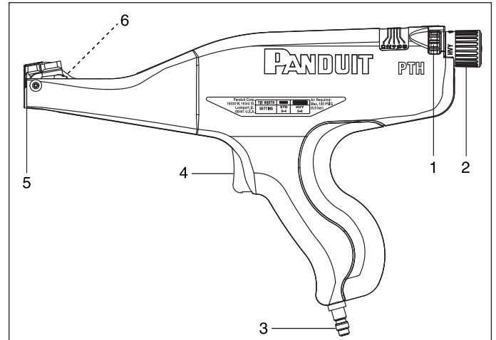
Attrezzo pneumatica PTH
