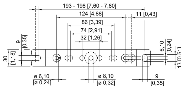
Montageschiene
