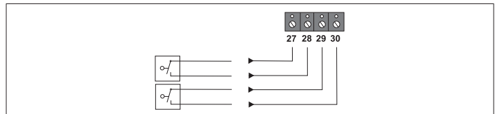
Abb. 30: Anschluss mit zwei Endschalter
