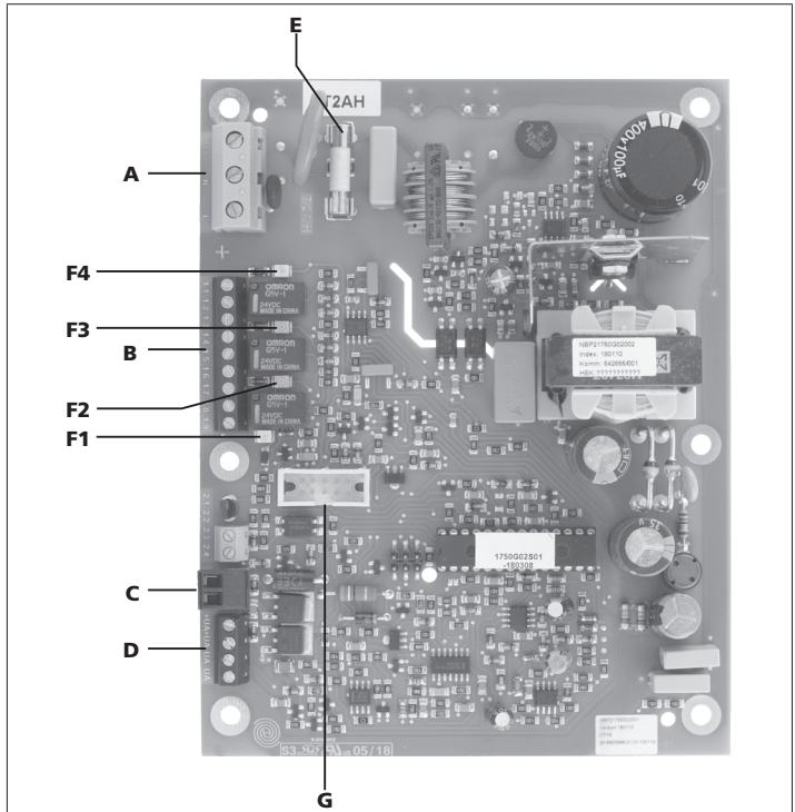
Abb. 13: Anschluss SVK 48
