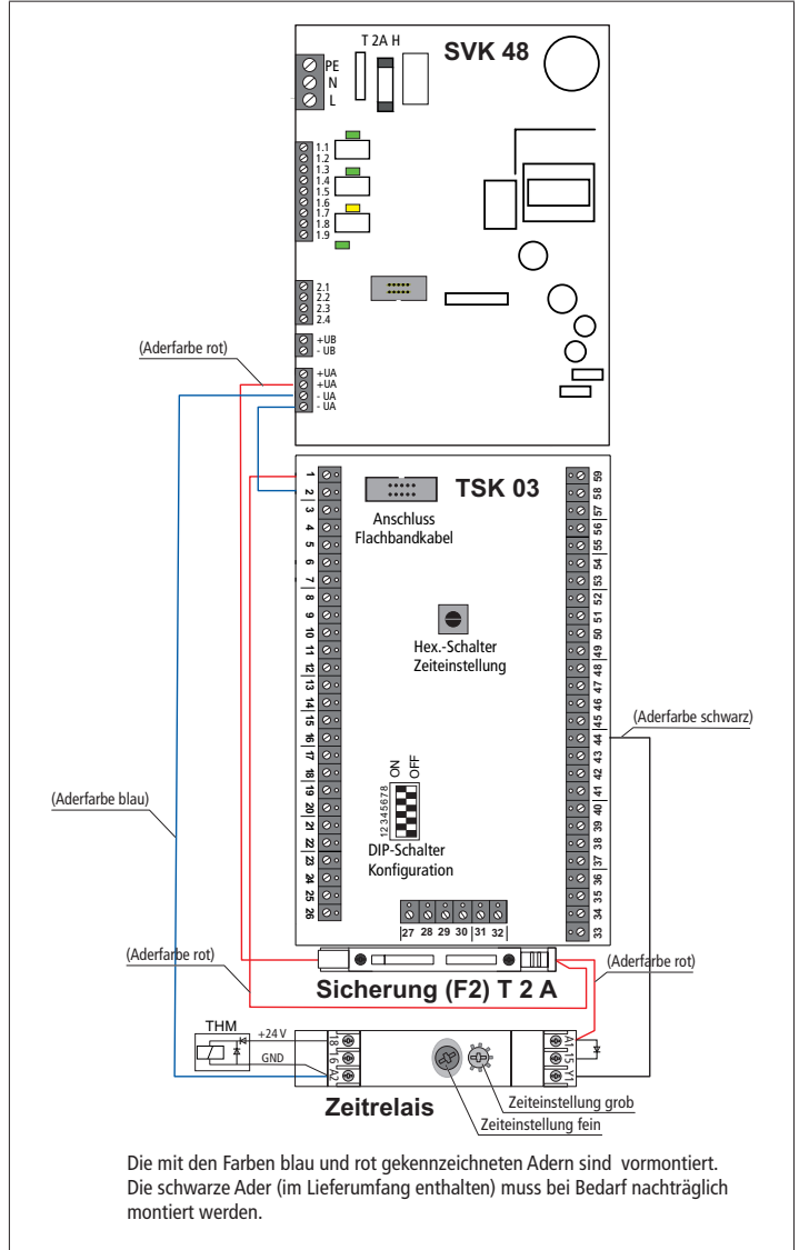
Abb. 07: Anschaltbeispiel für Klappensteuerung
