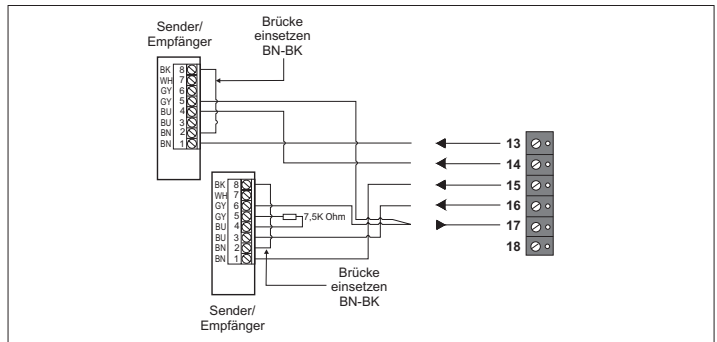
Abb. 21: Gruppenschaltung von 2 BRL-FSA/RLK 28-FC-55-Z/31/116
