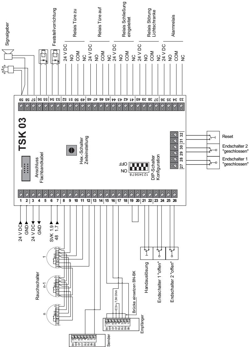
Abb. 14: Anschaltbeispiel der TSK 03 an einer Feststellanlage an bahngebundener Förderanlage
