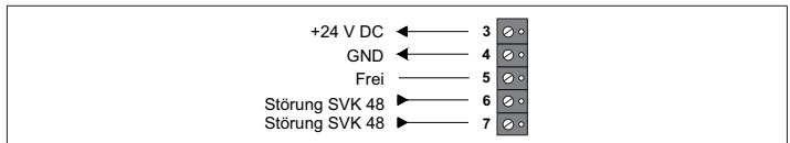
Abb. 16: Anschlüsse sind werkseitig vorverdrahtet
