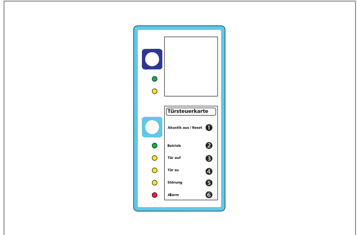
Abb. 03: Bedienfeld für die Türsteuercarte TSK 03
