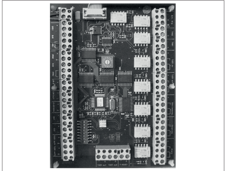
Abb. 05: Platine Türsteuerkarte TSK 03
