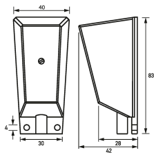
Maßzeichnung Gruppenansicht
