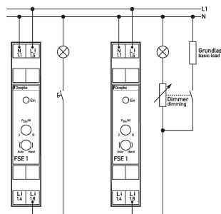
Anschlussschema
