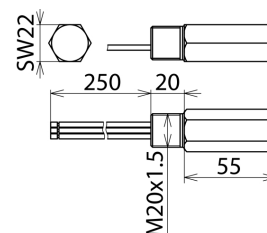
Maßbild DPI CD EXI 24 M
