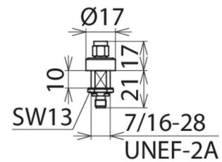
Maßbilder DGA G SMA
