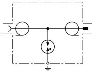
Prinzipialschaltbild DGA G SMA
