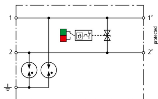
Principalschaltbild BCO CL2 BD HC10A 24
