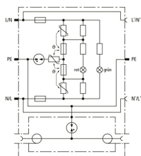
Principalschaltbild DPRO 230 TV
