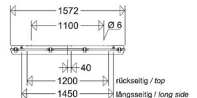
Zusätzliche Kabeleinführung (mit Presshaut) Additional entries (knock-outs)
