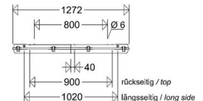
Zusätzliche Kabeleinführung (mit Presshaut) Additional entries (knock-outs)
