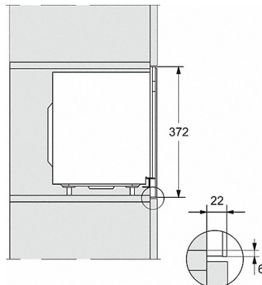
M22xxSC, Skizze
