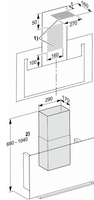
DADC 9000 (Skizze)
