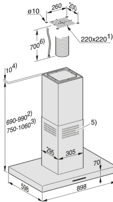
DA 410-6, DA 4208 D, DA 4208 D EXTA, DA 6396 D, DA 6596 D, PUR 98 D (Skizze)
