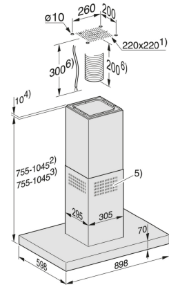
DA 420 V-6, DA 4208 VD (Skizze)
