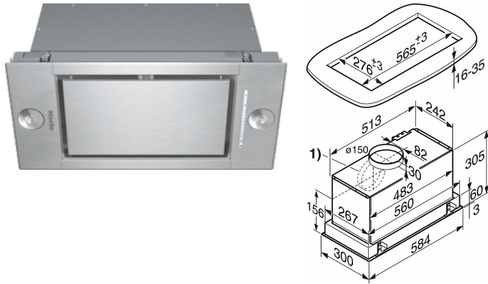
DA 2668 Lüfterbaustein (Skizze)
