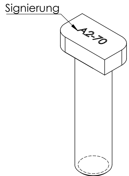
Isometrie M 2:1
