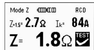
Bild 3.22 Impedanz hinter einem FI (detailliert)
