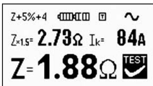
Bild 3.19 Gemessene Impedanz + Messabweichung
