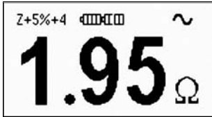
Bild 3.17 Impedanz + Messabweichung
