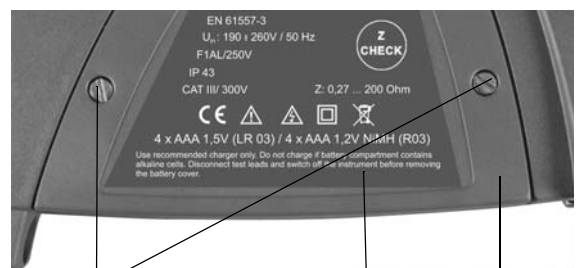
Bild 2.2 Detail der Rückwand mit Batteriefachdeckel
